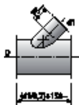
Abzweiger 45° Té 45°
