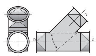
Abzweiger 45° mit Umlenkklappe (Betriebsdruck max. +/- 3'000 Pa) Clapet déflecteur 45° (Pression de service max. +/- 3'000 Pa)
