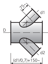
Kreuzstück 45° Croix 45° L = (d3 : 0.7) + ~150
