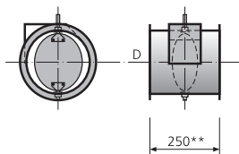
Regulierklappe mit Konsole Clapet de réglage avec support
