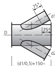
Kreuzstück 30° Croix 30° L = (d3 : 0.5) + ~150
