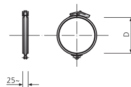
Spannring für EB (mit Dichtung) Bride pour EB avec joint
