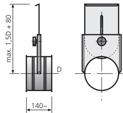
Absperrschieber Registre
