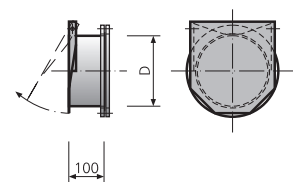
Rückschlagklappe (einfache Ausführung) Clapet anti-retour (Exécution simple)
