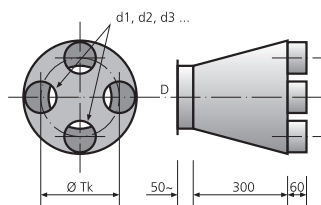
Absaug-Glocke Collecteur d'aspiration
