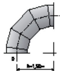
Segmentbogen, R = 1.5 d1 Coude à segments, R = 1.5 d1
