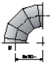
Segmentbogen, R = 1 d1 Coude à segments, R = 1 d1
