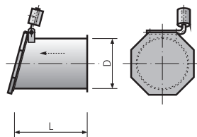
Rückschlagklappe für horizontalen Einbau Clapet anti-retour pour montage horizontale
