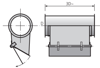
Klotzabscheider Séparateur
